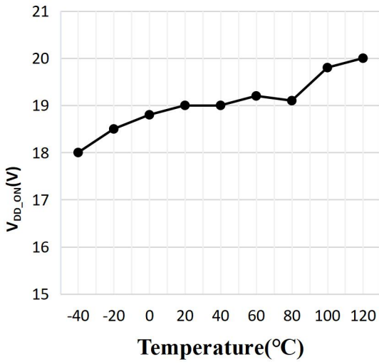
V_{DD\_ON} vs Tem
